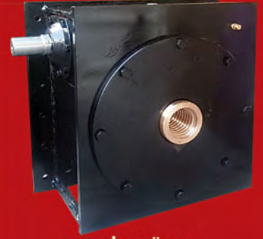
ÇELİK GÖVDE BARAJ KAPAK REDÜKTÖRÜ STEEL CENTRIC DAM SHUTTER REDUCER
