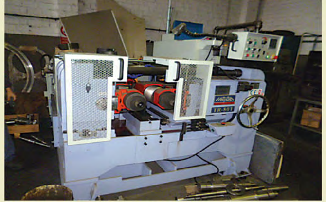
OVALAMA / CRUMBLING 80 TON
