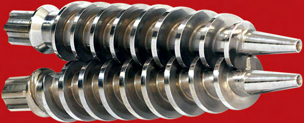
MANGAL KÖMÜRÜ SIKIŞTIRMA HELEZONU / CHARCOAL COMPRESSION SPIRAL
